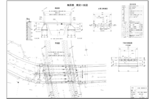
橋梁一般図
